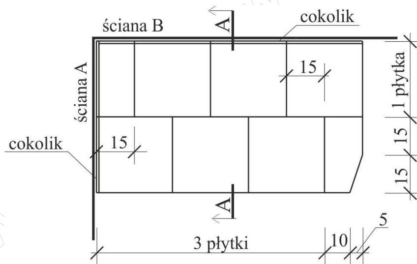
Rysunek 1. Usytuowanie posadzki z cokolikiem na podłodze
