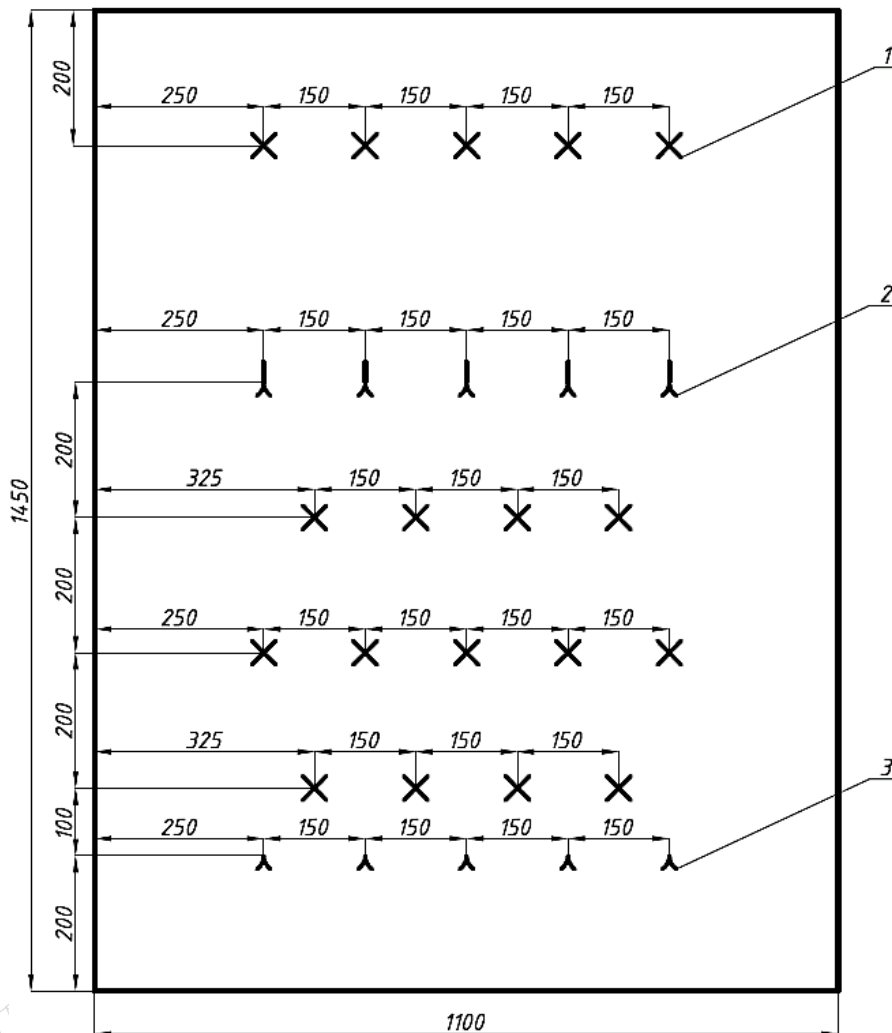
Schemat 2. Siatka pikowania i rozmieszczenie wieszaków 1 – guzik, 2 – wieszak duży, 3 – wieszak mały
