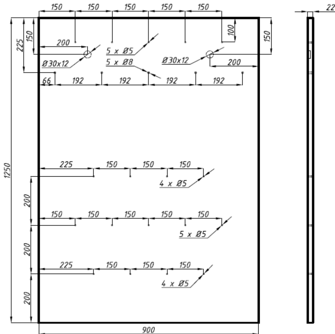
Schemat 1. Rozmieszczenie otworów na płycie panelu
