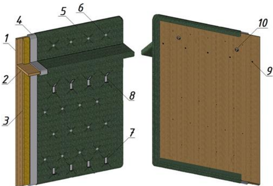
Ilustracja 2. Konstrukcja panelu wieszakowego tapicerowanego
