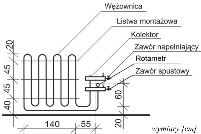
Rysunek. Schemat ogrzewania płaszczyznowego ściennego
