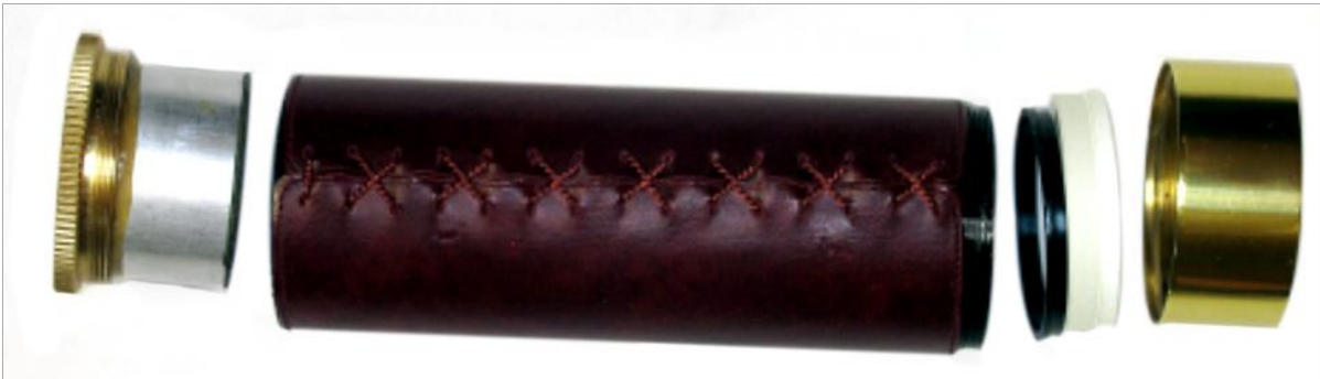
Rysunek 4. Obiektyw lunety kapitańskiej 12 x 30 w rozbiorze na części
