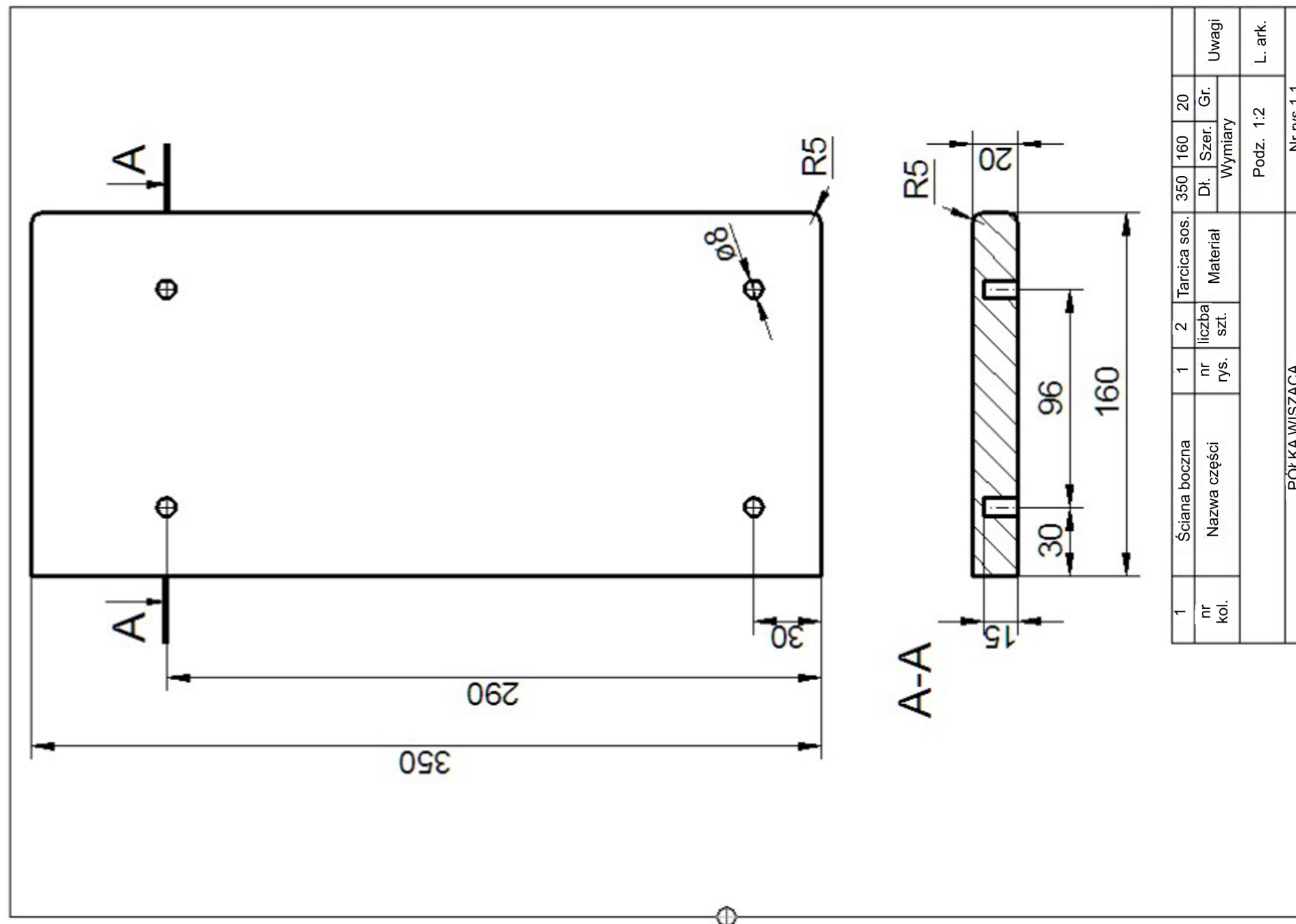
Rysunek 3. Ściana boczna
