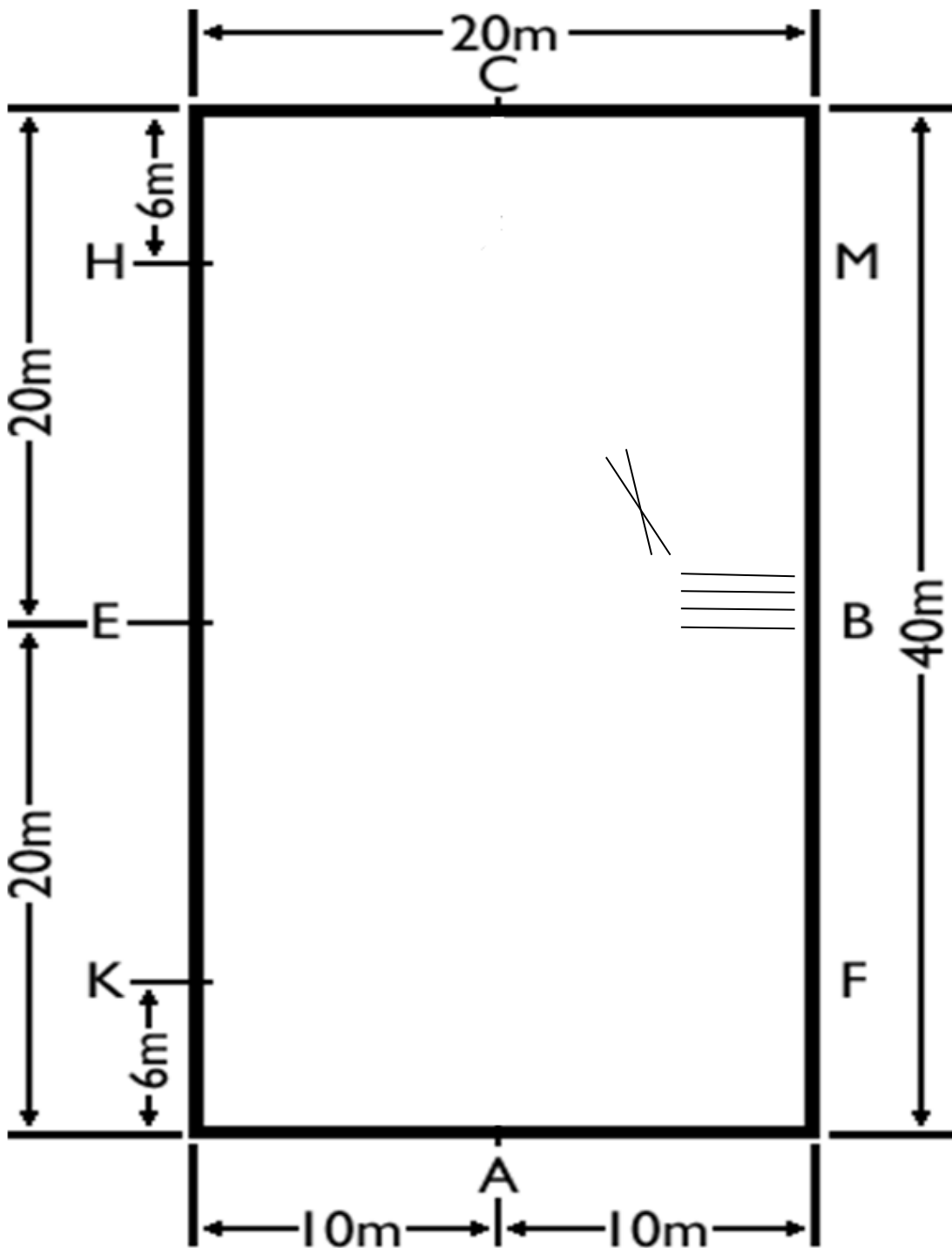
Schemat czworoboka:
