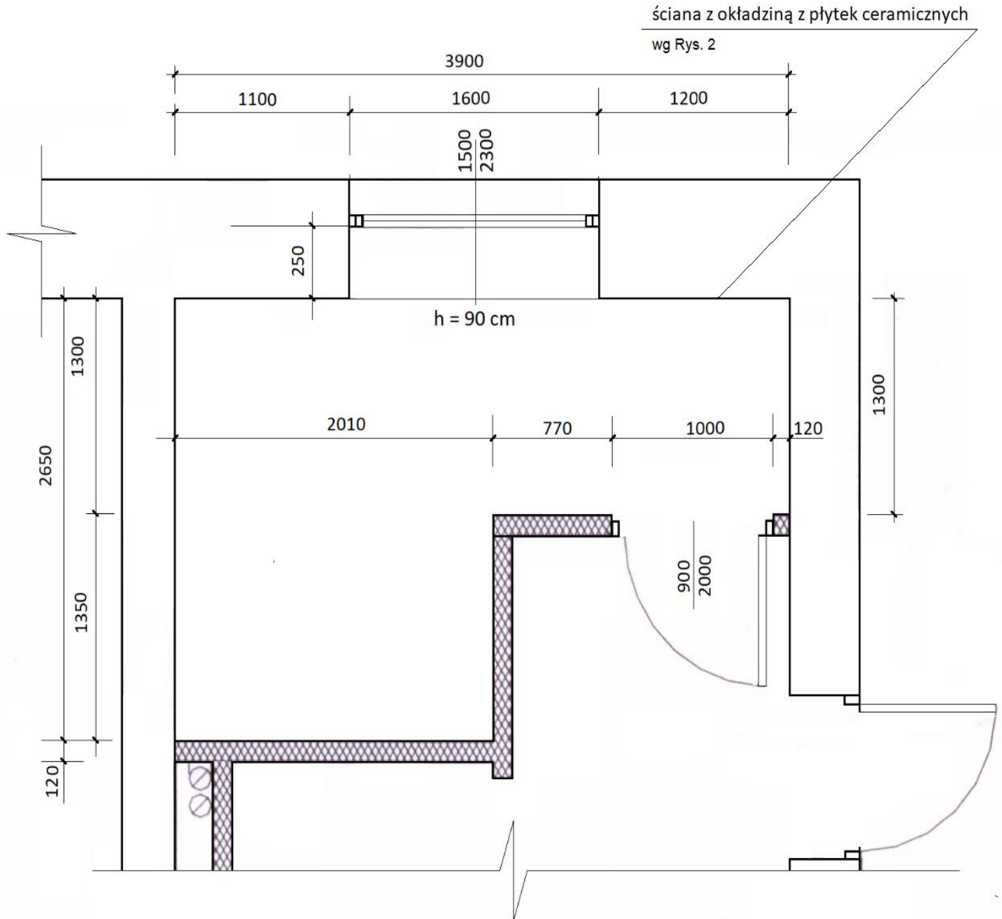
Rysunek 1. Rzut łazienki
