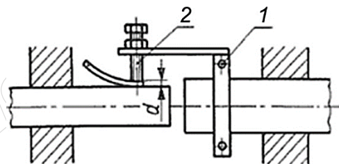
1 - zacisk, 2 śruba
