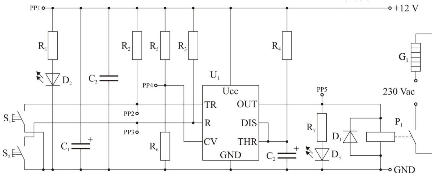
Rys. 1. Włącznik czasowy z zaznaczonymi punktami pomiarowymi
