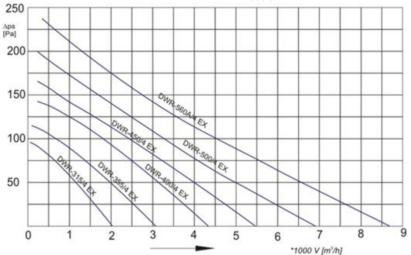
Charakterystyki aerodynamiczne
