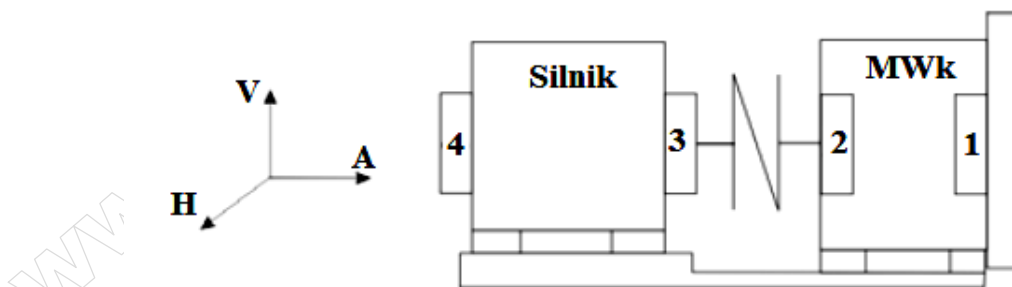
Schemat z punktami pomiarowymi na obudowach łożysk
