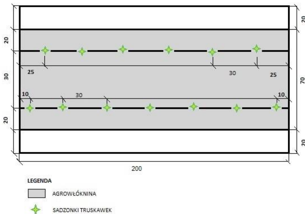
Rysunek 1: Schemat sadzenia sadzonek truskawek w dwóch rzędach
