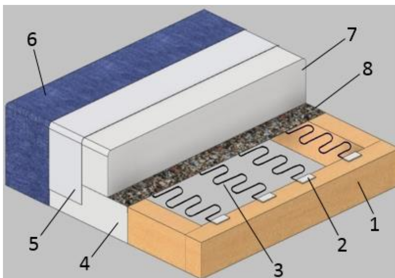
Rysunek 1. Przekrój siedziska pufu
