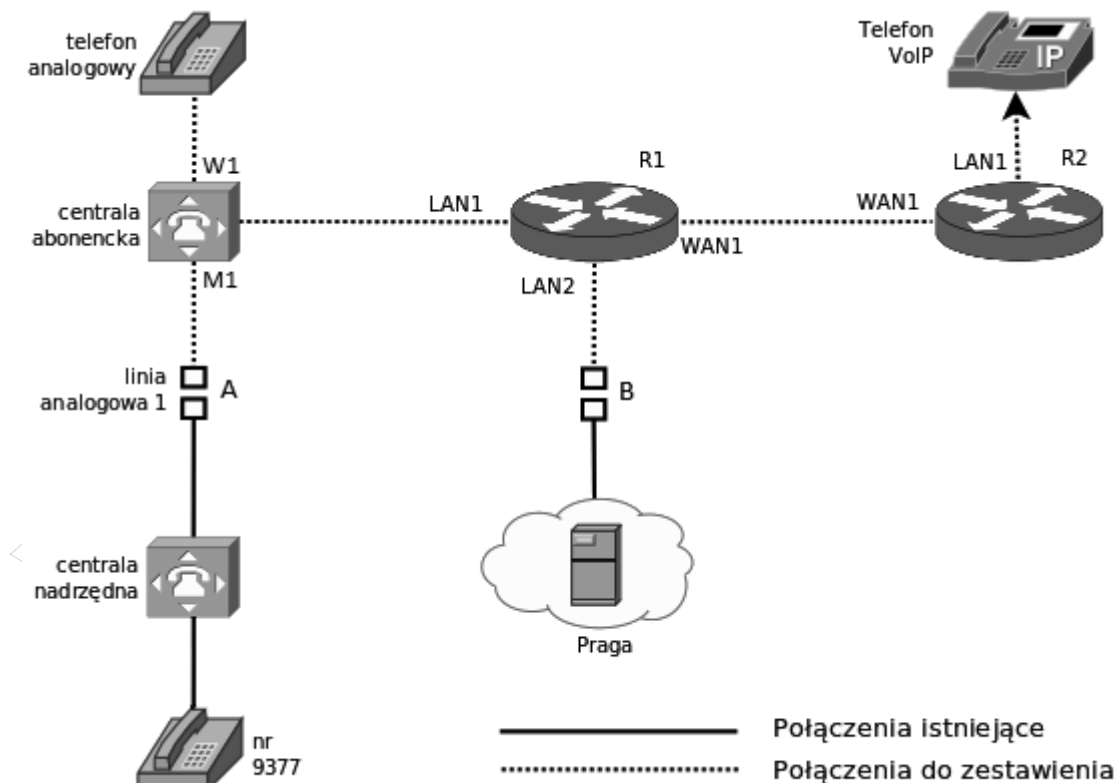
Rys.1. Schemat usytuowania urządzeń w sieci teleinformatycznej
