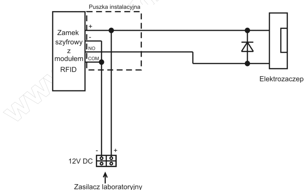
Rysunek 1. Schemat montażowy instalacji systemu kontroli dostępu.
