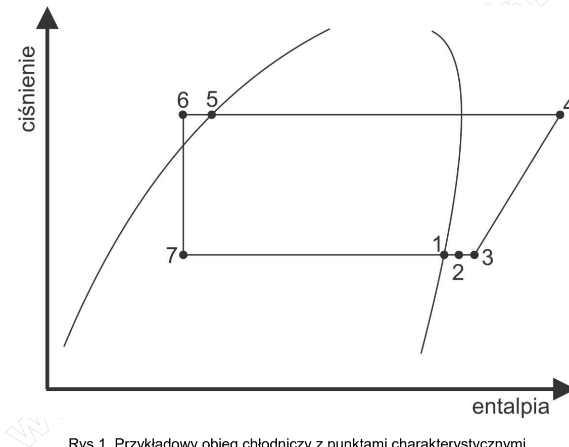
Rys.1. Przykładowy obieg chłodniczy z punktami charakterystycznymi
