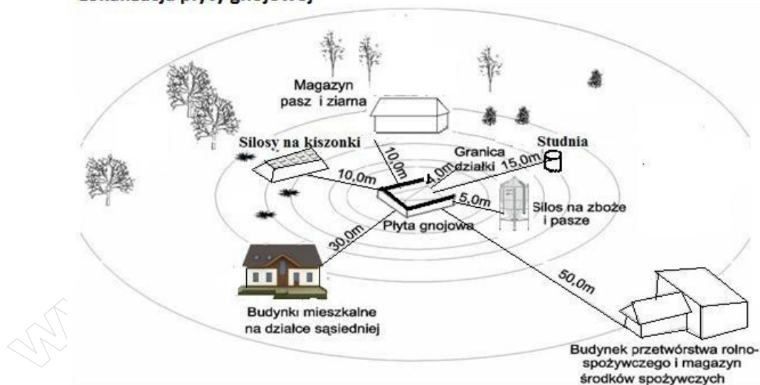
Lokalizacja płyty gnojowej
