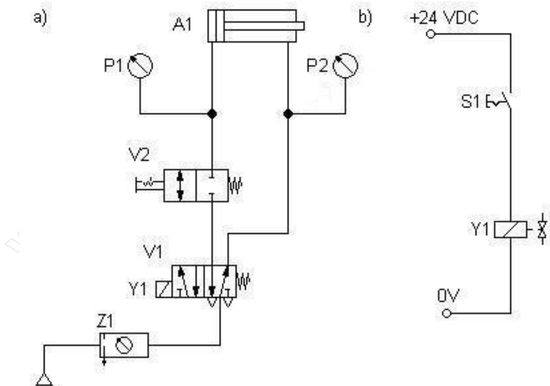
Rysunek 1. Schemat połączeń układu do sprawdzania działania siłownika pneumatycznego: a) pneumatyczny; b) elektryczny
