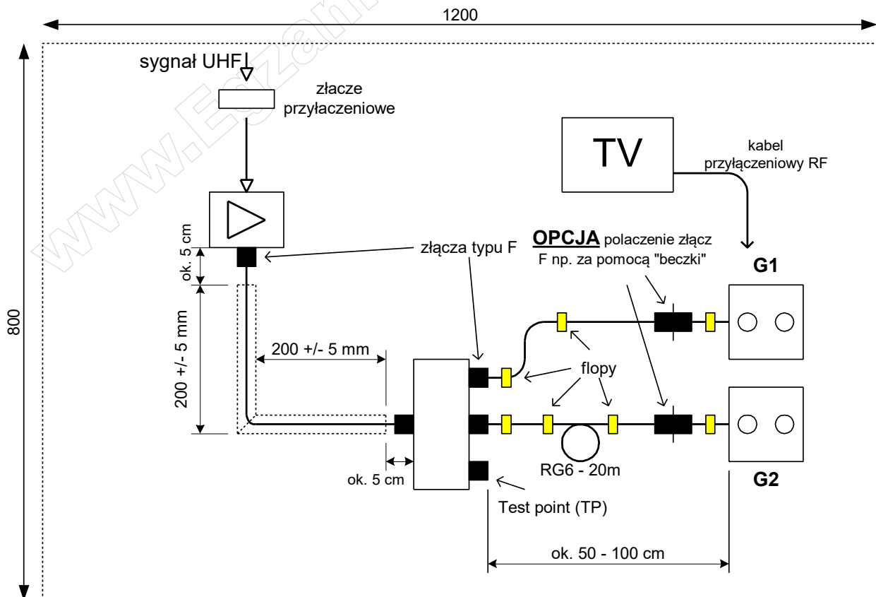
Rysunek 1. Schemat instalacji
