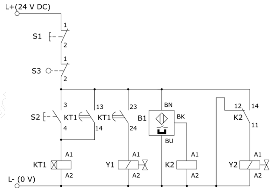
Rysunek 2. Schematy połączeń elektrycznych układu do zmontowania
