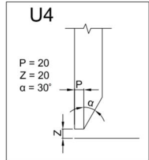
Rysunek 2. Zakończenia usztywnień
