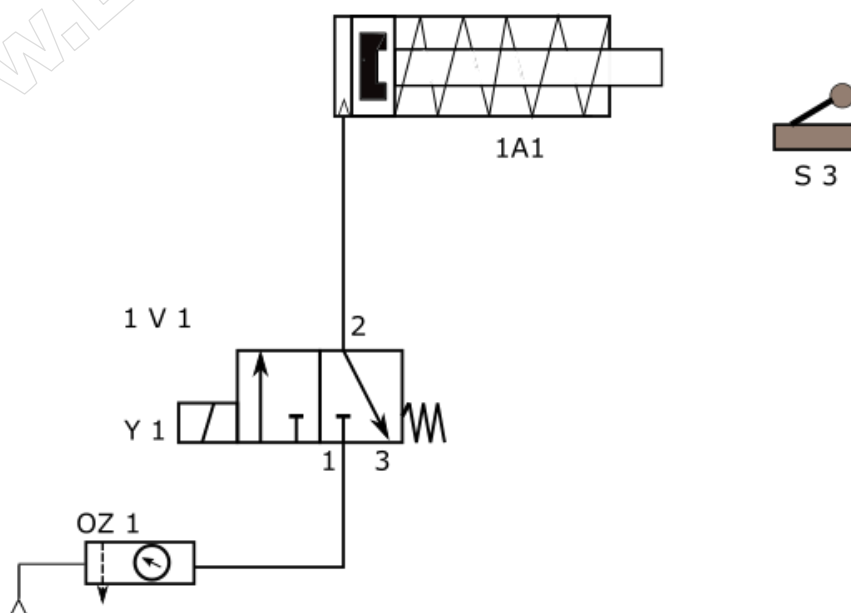
Rysunek 3. Schemat pneumatyczny układu sterowania silownikiem
