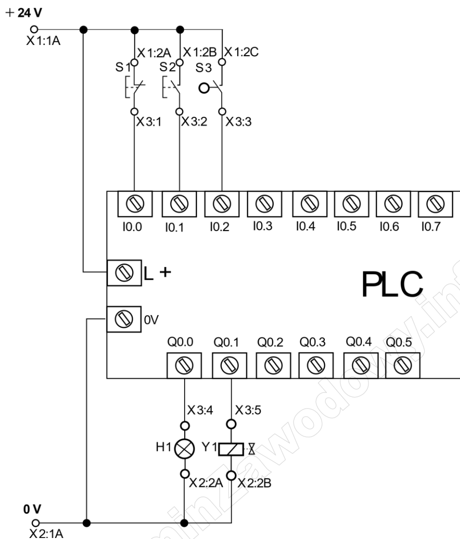
Rysunek 2. Schemat elektryczny układu sterowania silownikiem
