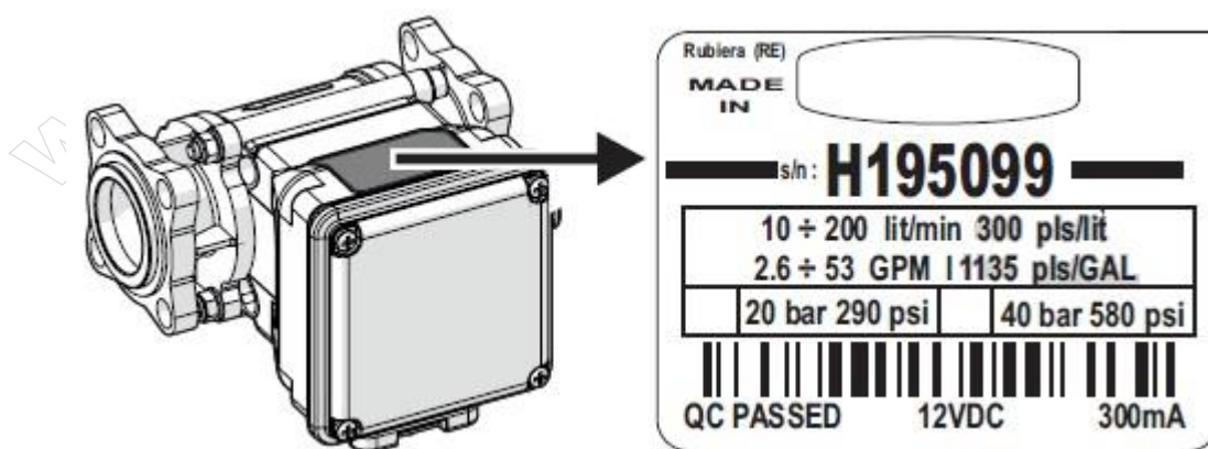
Rysunek 1. Przepływomierz
