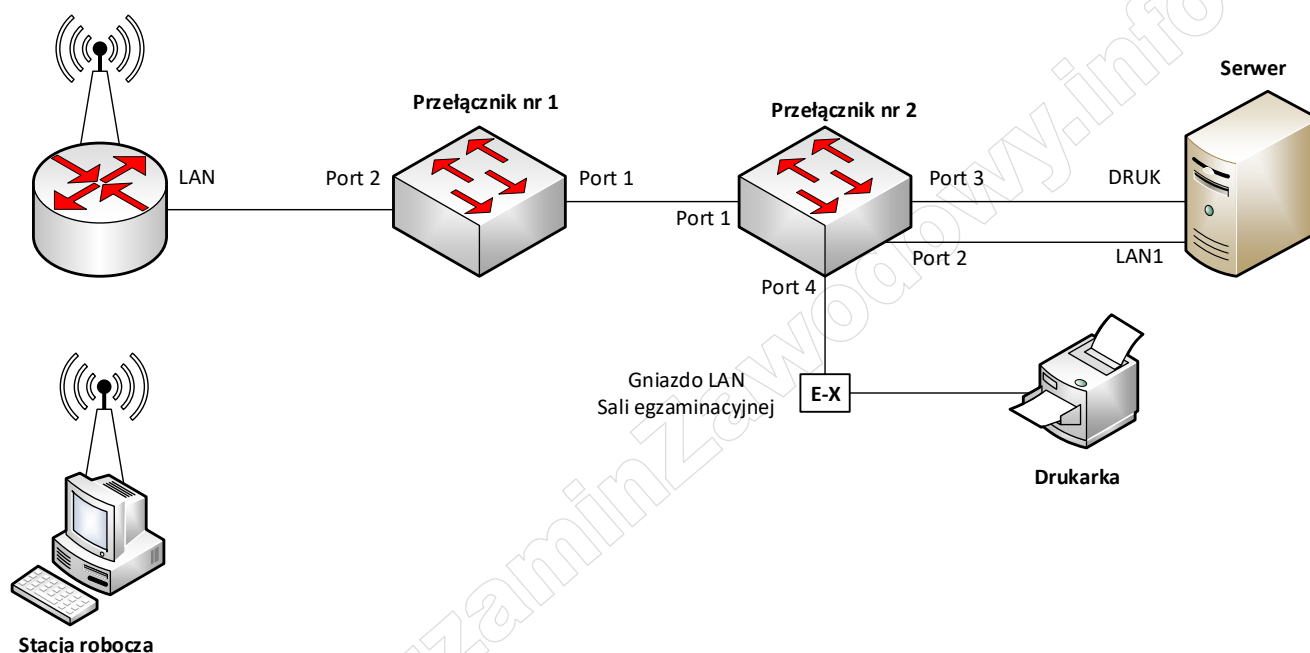
Schemat podłączeń urządzeń w sieci lokalnej
