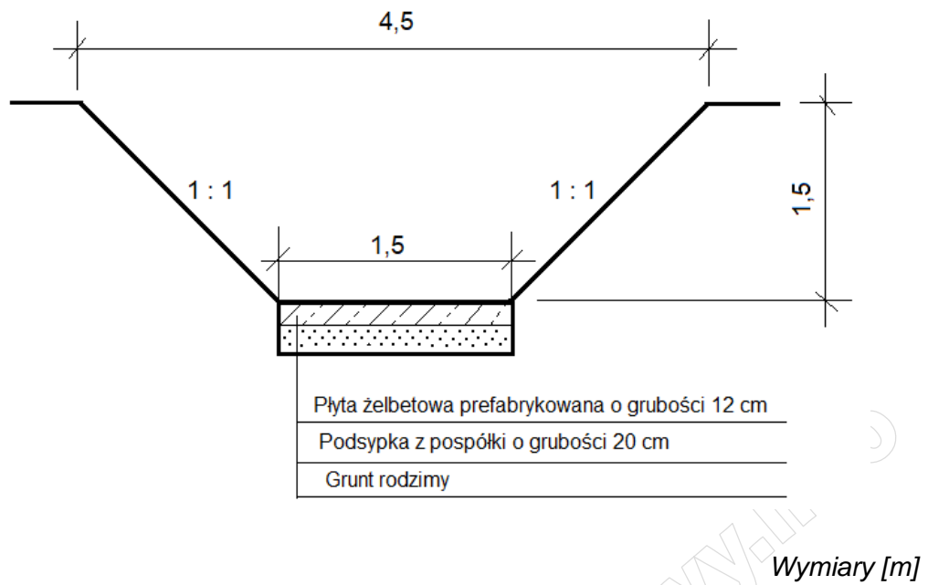
Rysunek 1. Przekrój poprzeczny wykopu i umocnienia dna wykopu
