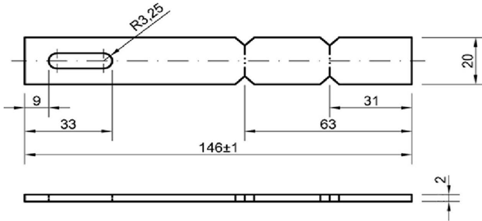
Rysunek 2. Okucie budowlane
