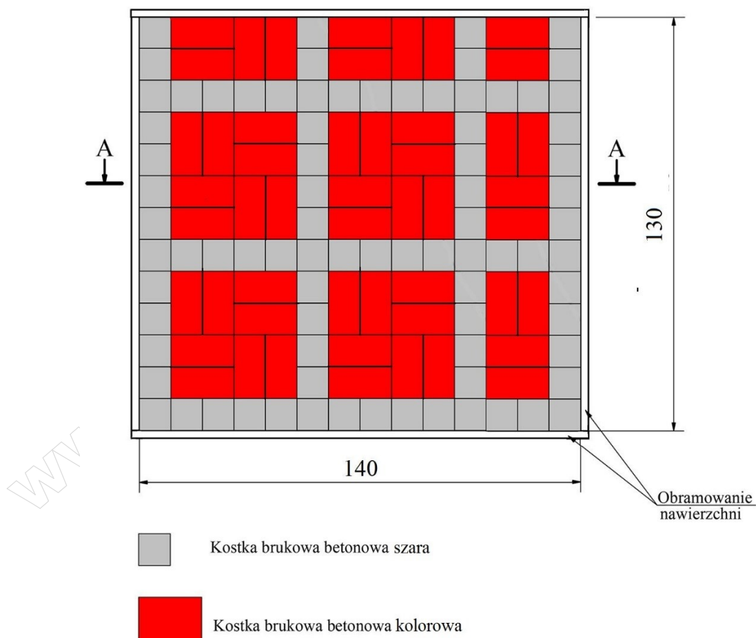
Rysunek 1. Rzut poziomy fragmentu nawierzchni do ułożenia
