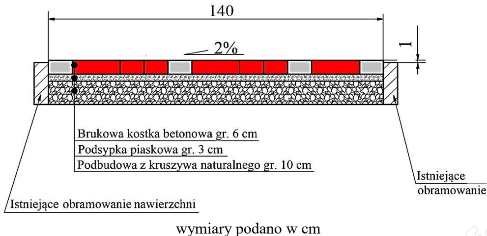
Rysunek 2. Przekrój poprzeczny nawierzchni z betonowej kostki brukowej
