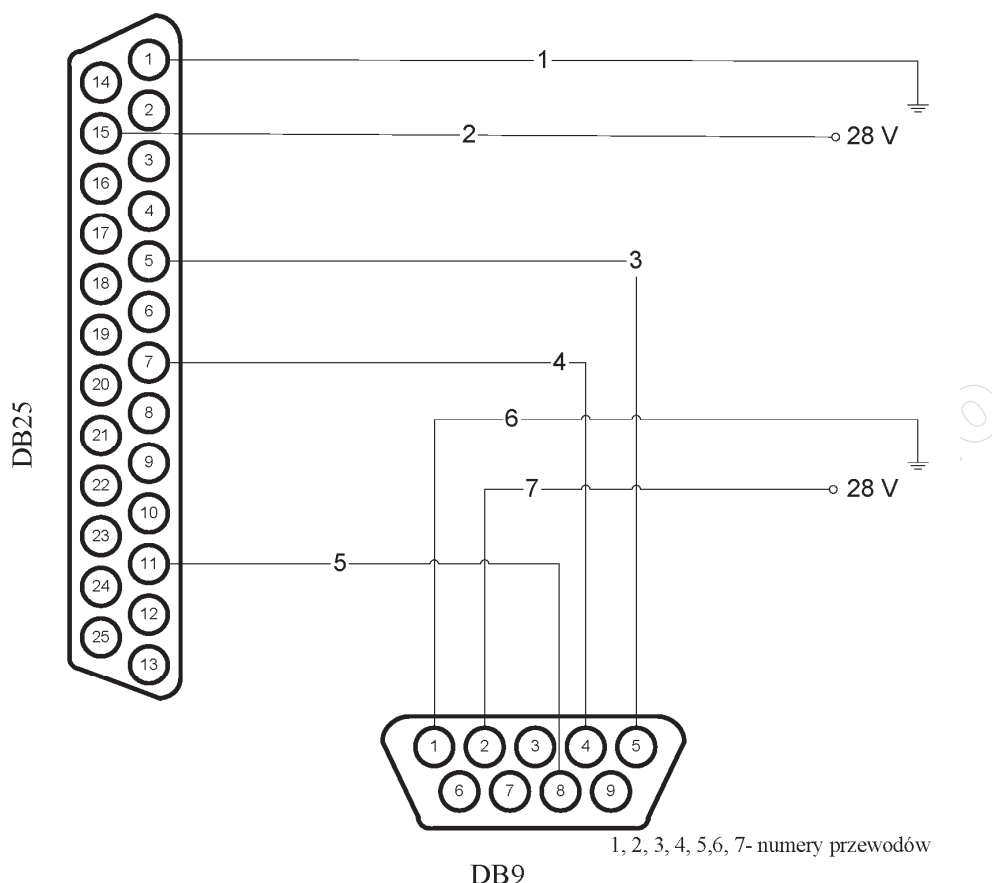
Rys. 6. Schemat wiązki
