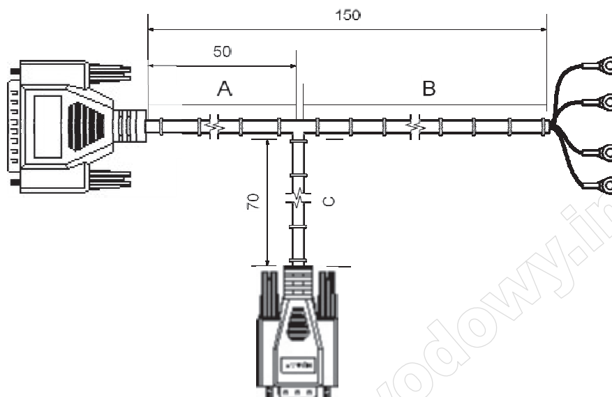
Rys.1. Wiązka elektryczna w widoku (wymiarów podano w cm)
